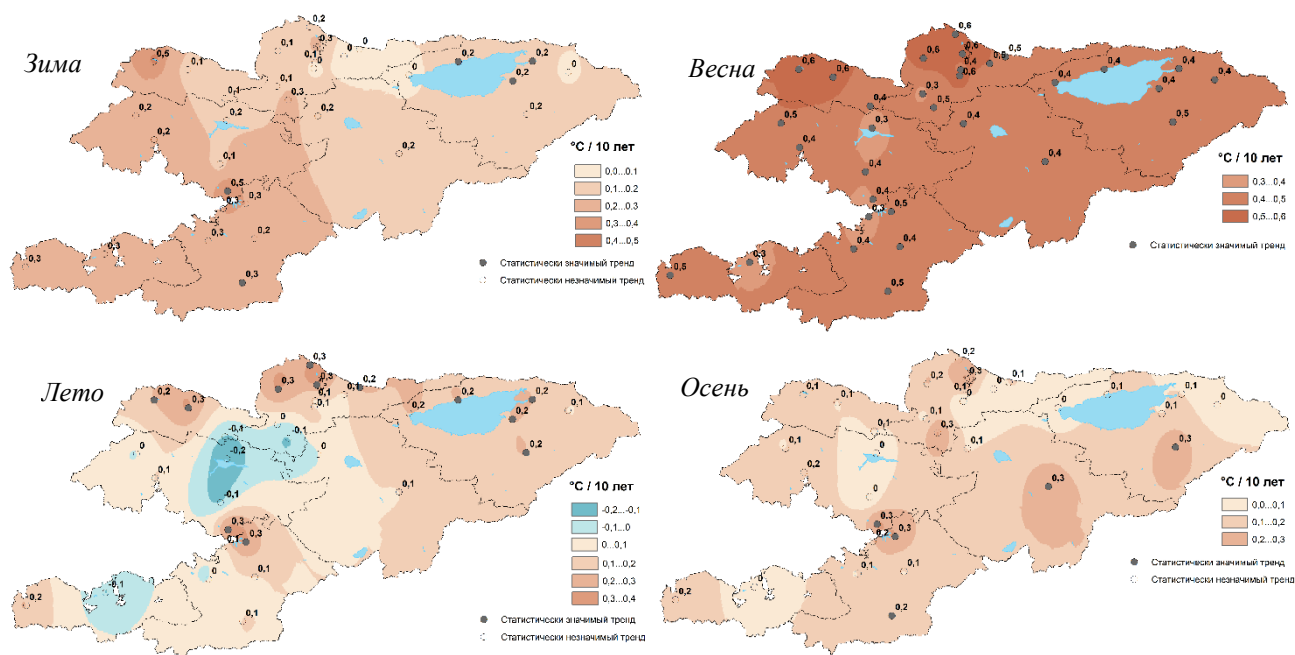
Рисунок 2.3 – Пространственное распределение значений коэффициента линейного тренда средней сезонной температуры приземного воздуха ( ^{\circ}\text{C}/10 лет), рассчитанного по данным наблюдений за период 1976 - 2019 гг.
