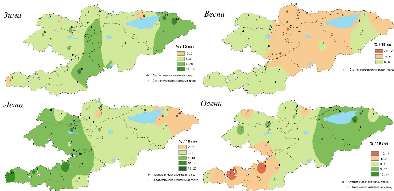
Рисунок 2.8 – Пространственное распределение коэффициента линейного тренда аномалий сезонных сумм осадков (%/10 лет), рассчитанных за период 1976 - 2019 гг.
