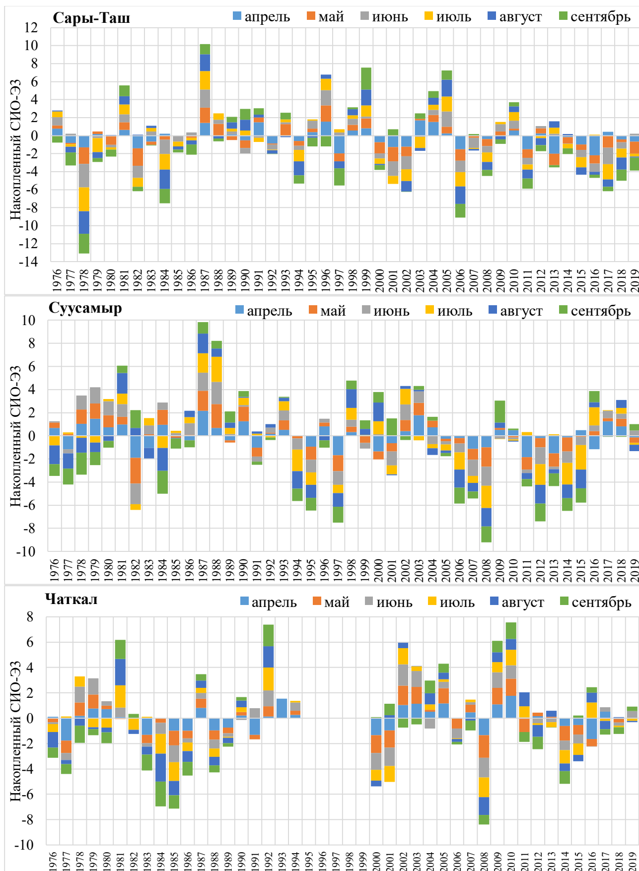
Рисунок 4.8. – временное распределение накопленного за вегетационный период СИО-ЭЗ (продолжение)
